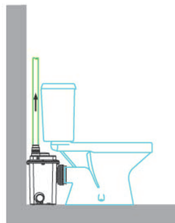
马桶后安装
