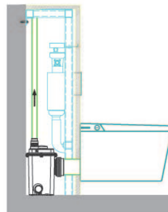
假墙内隐蔽安装
