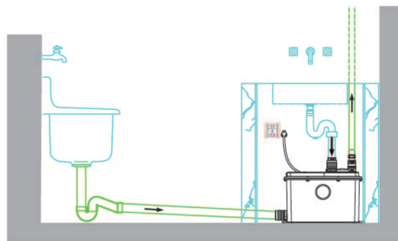
侧面进水安装
